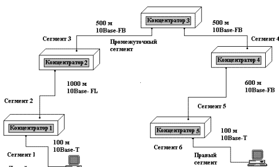
Рисунок 1. Пример сети Ethernet
